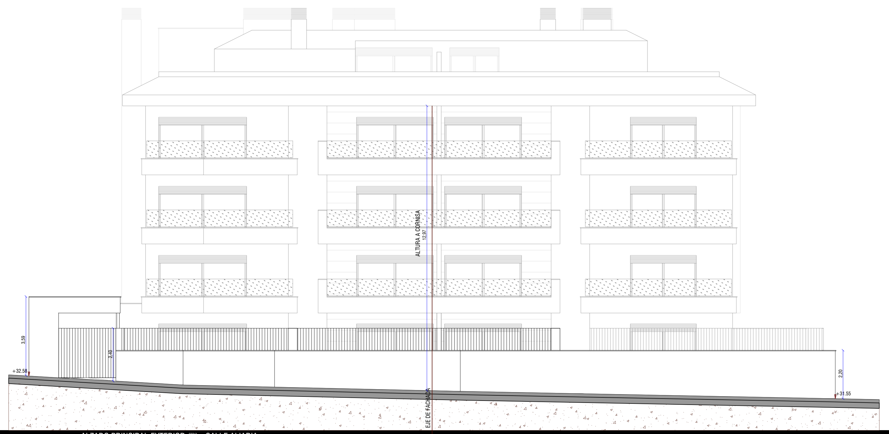
ALZADO PRINCIPAL EXTERIOR (H) - CALLE ALIARIA
