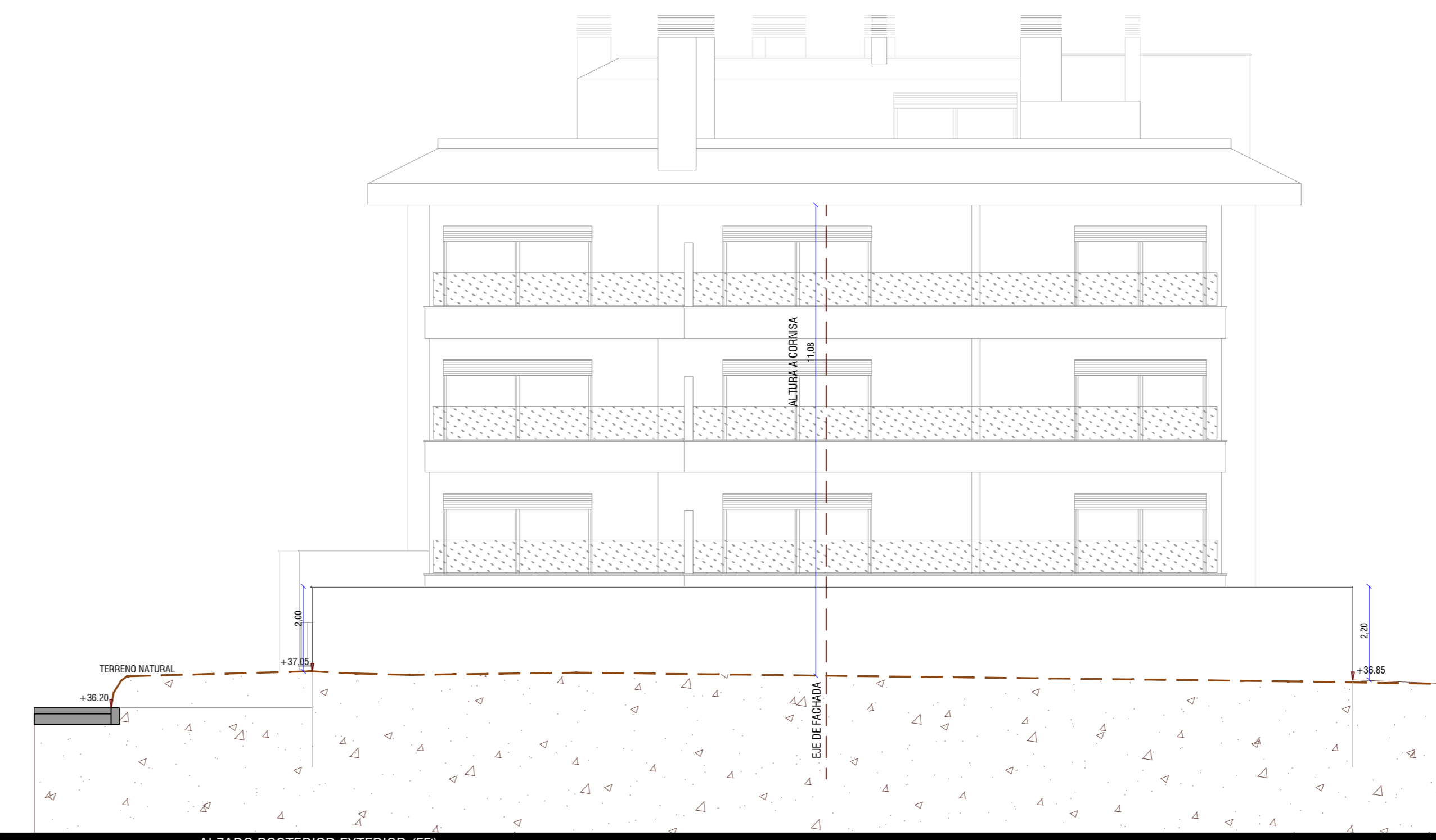
ALZADO POSTERIOR EXTERIOR (FF)
