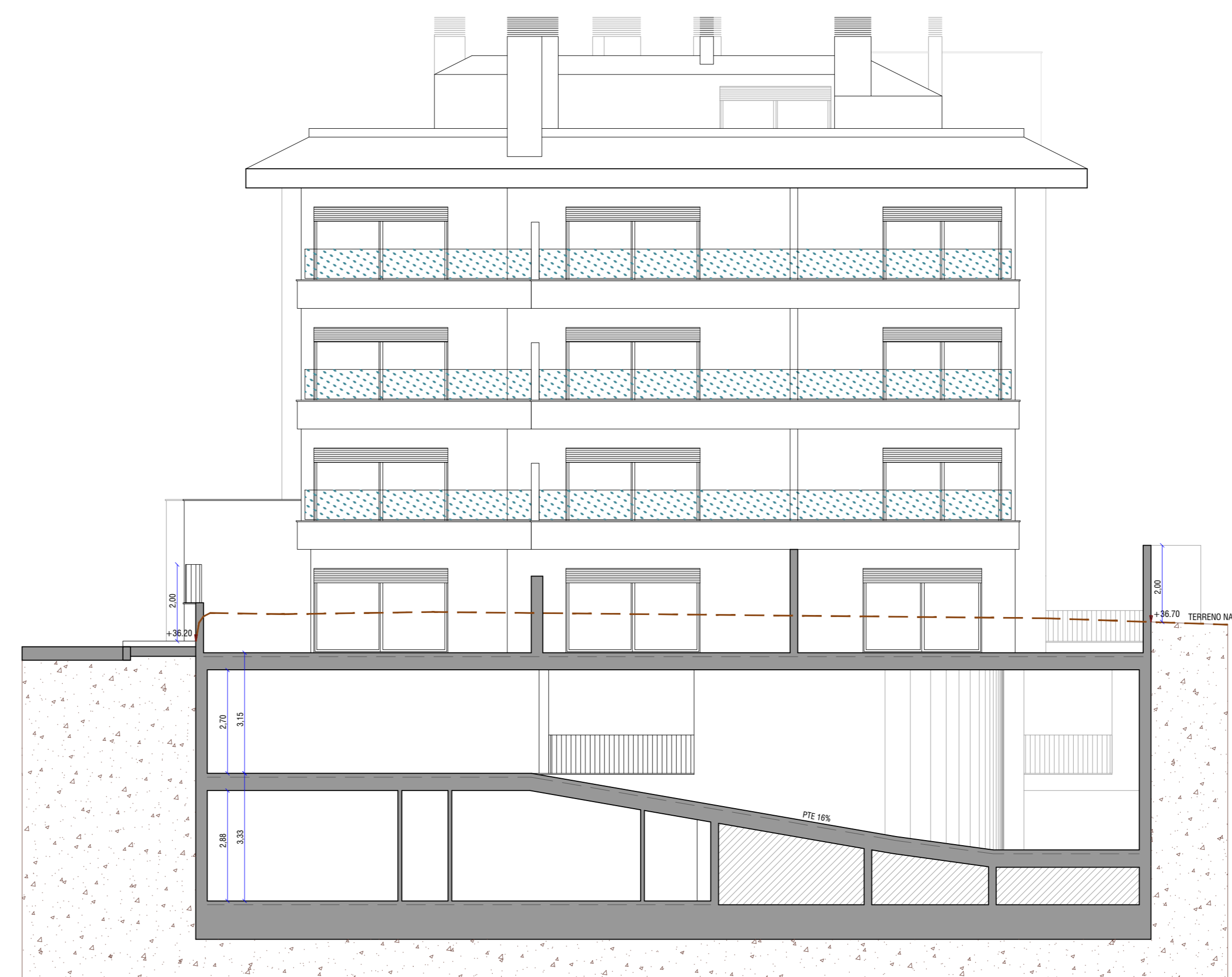
ALZADO POSTERIOR INTERIOR (GG)
