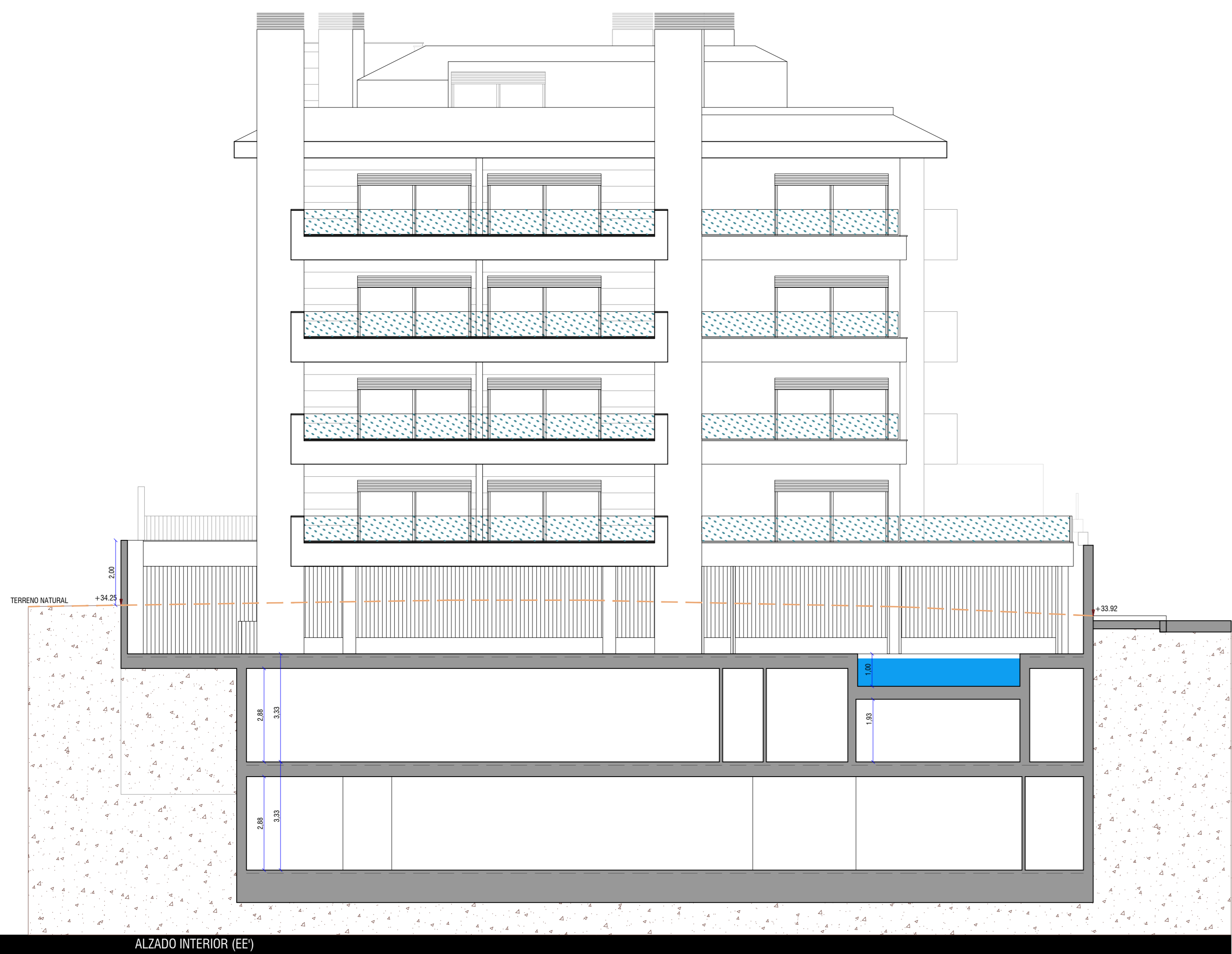
ALZADO INTERIOR (EE)
