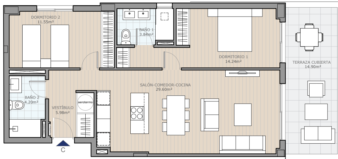
BLOQUE 2 - PLANTA PRIMERA - VIVIENDA C
