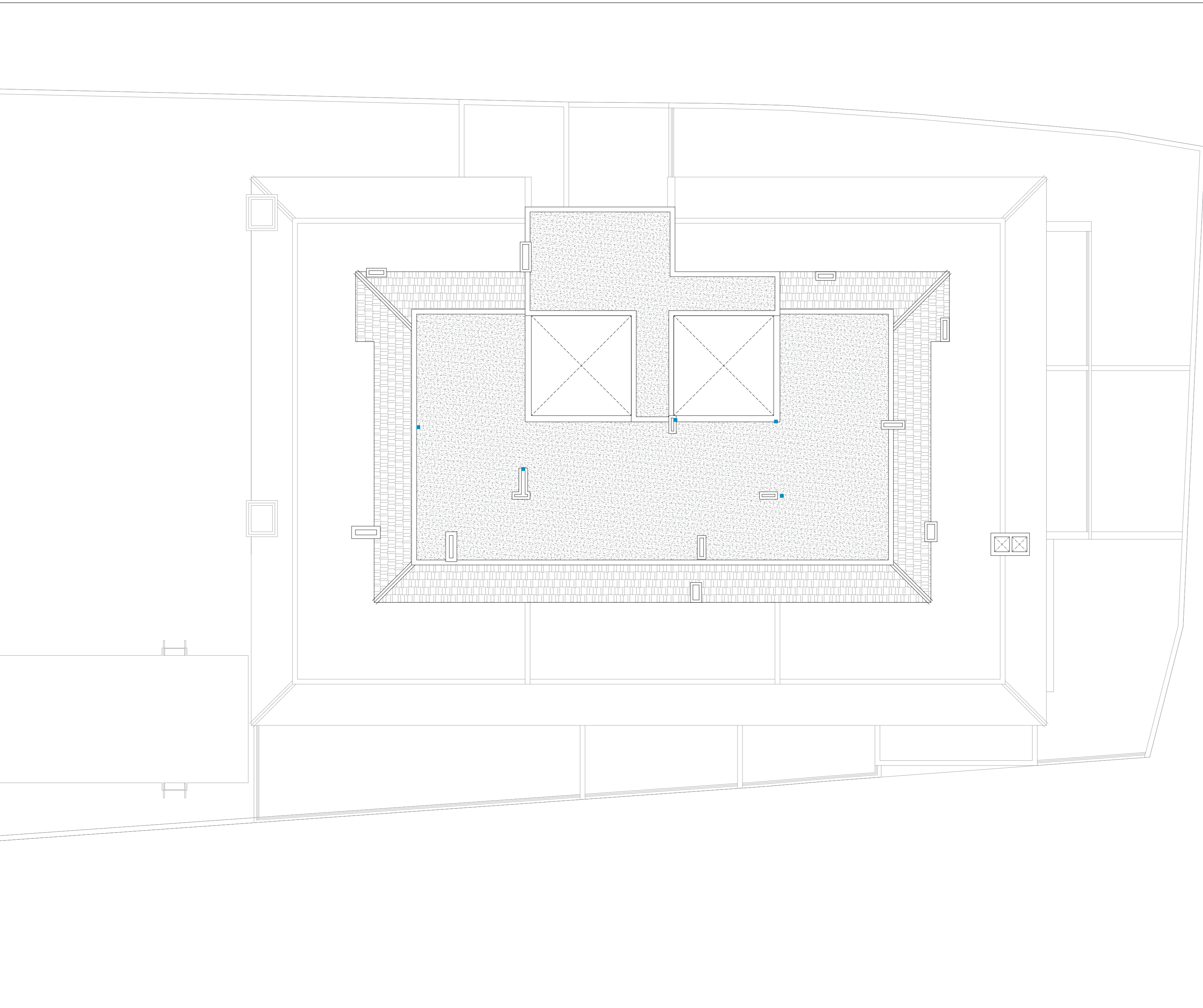
PLANTA CUBIERTAS - BLOQUE 2 (NIVEL 51,75 m)
