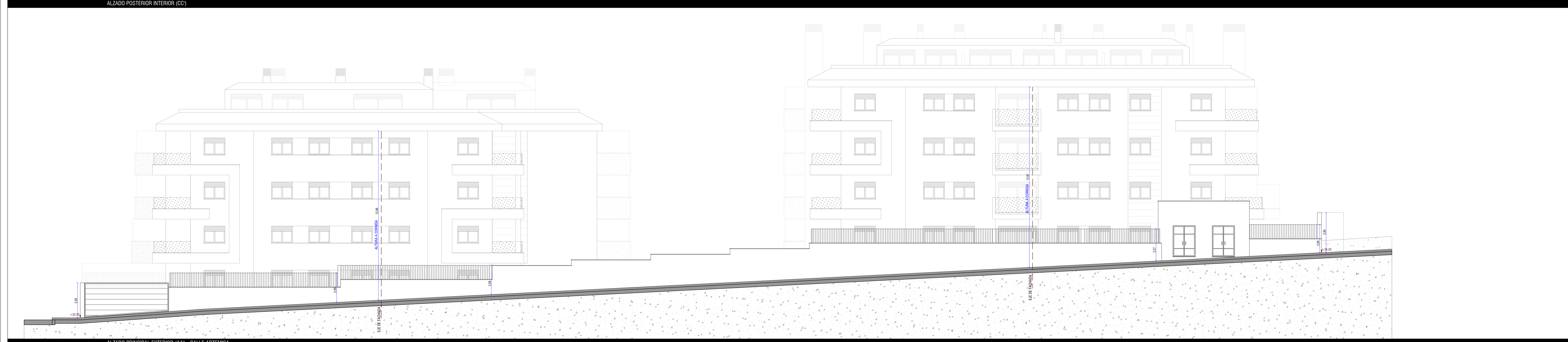
ALZADO PRINCIPAL EXTERIOR (AA) - CALLE ARTEMISA
