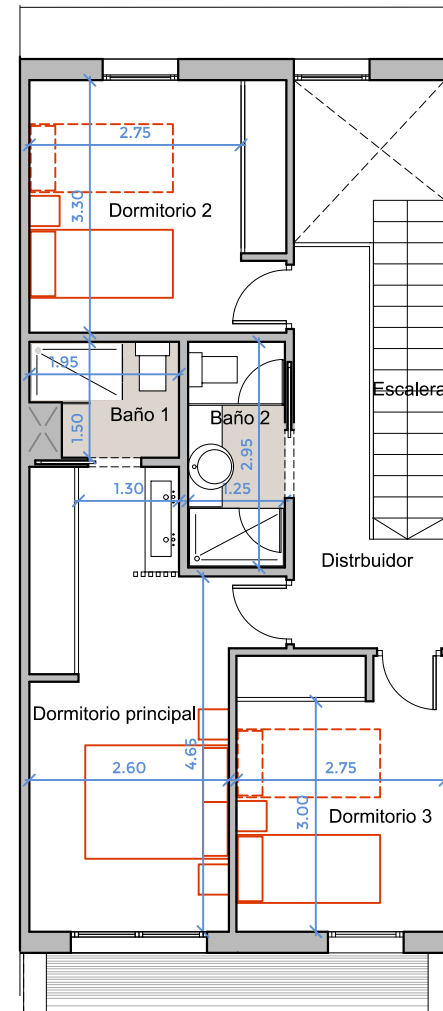
PLANTA PRIMERA
