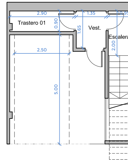
PLANTA SÓTANO
