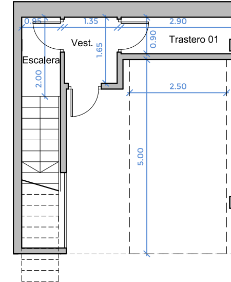
PLANTA SÓTANO
