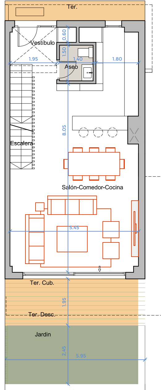
PLANTA BAJA
