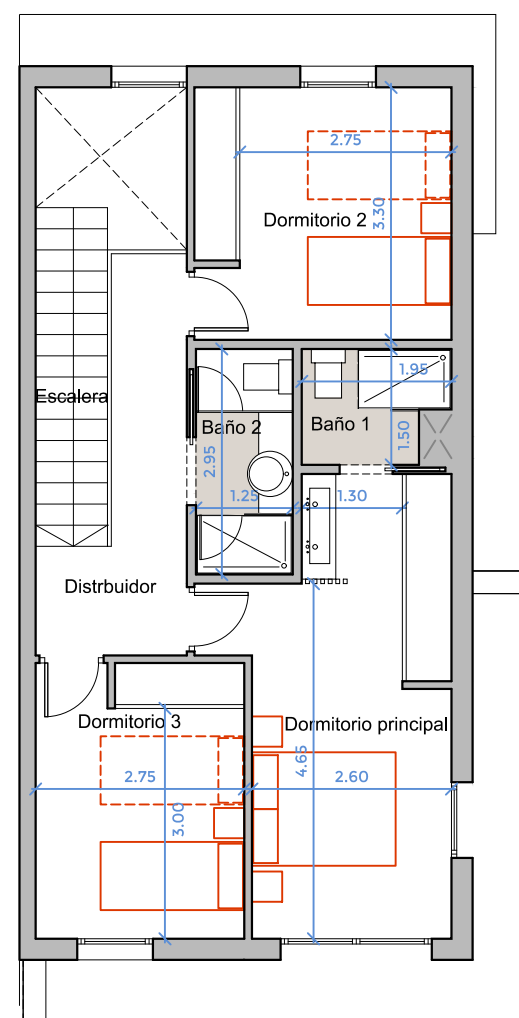
PLANTA PRIMERA
