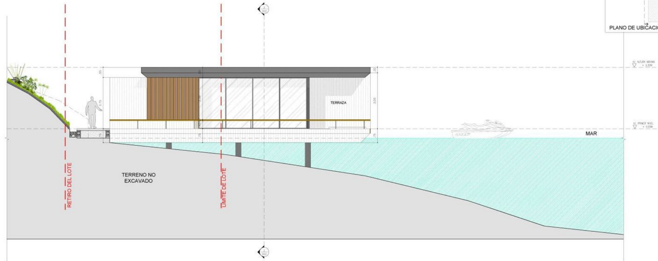
1 SECCIÓN LONGITUDINAL 1:50
