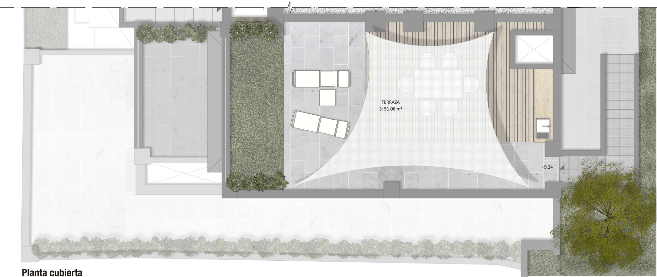
Planta cubierta
