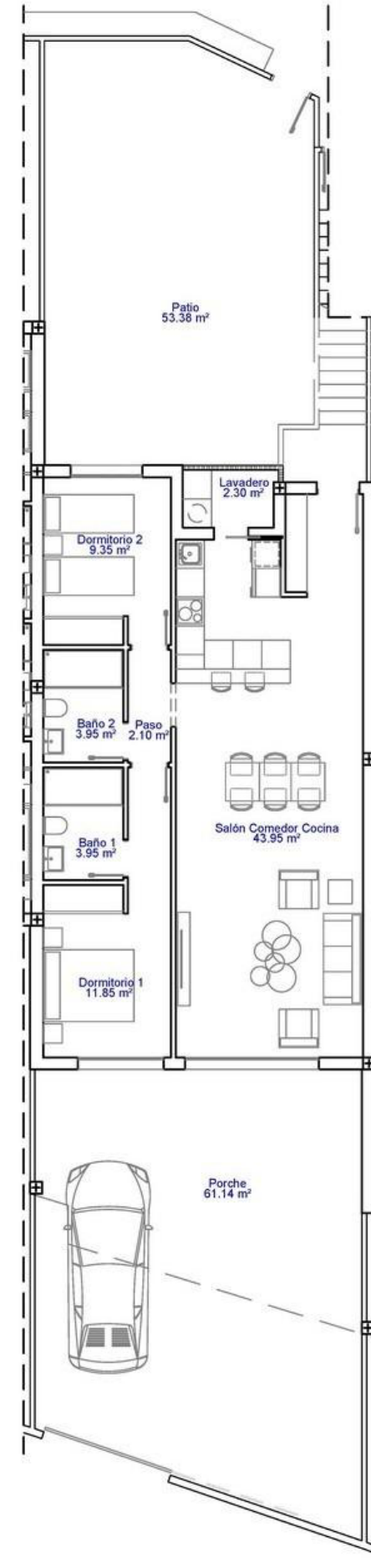
Planta Baja E:1/150
