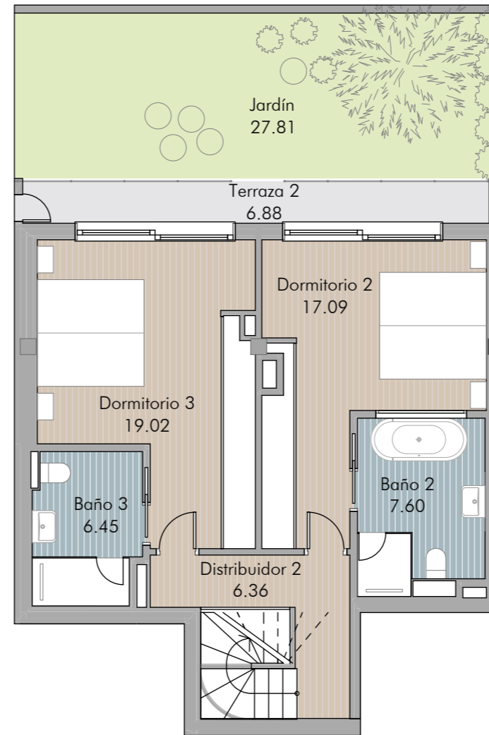
PLANTA SEGUNDA
