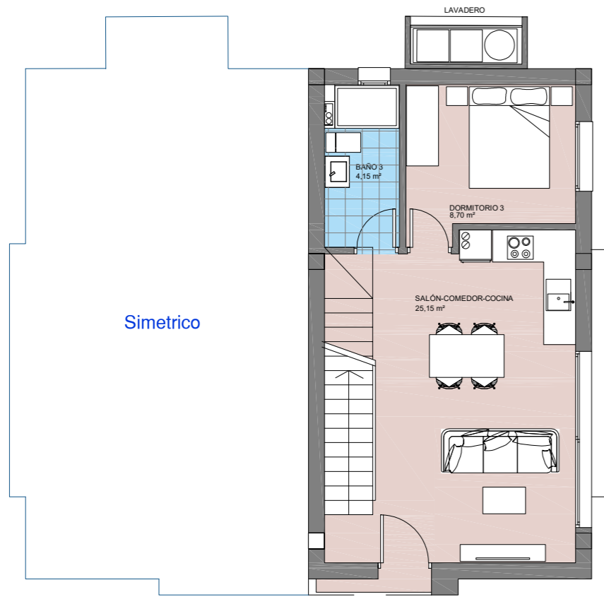
PLANTA BAJA
