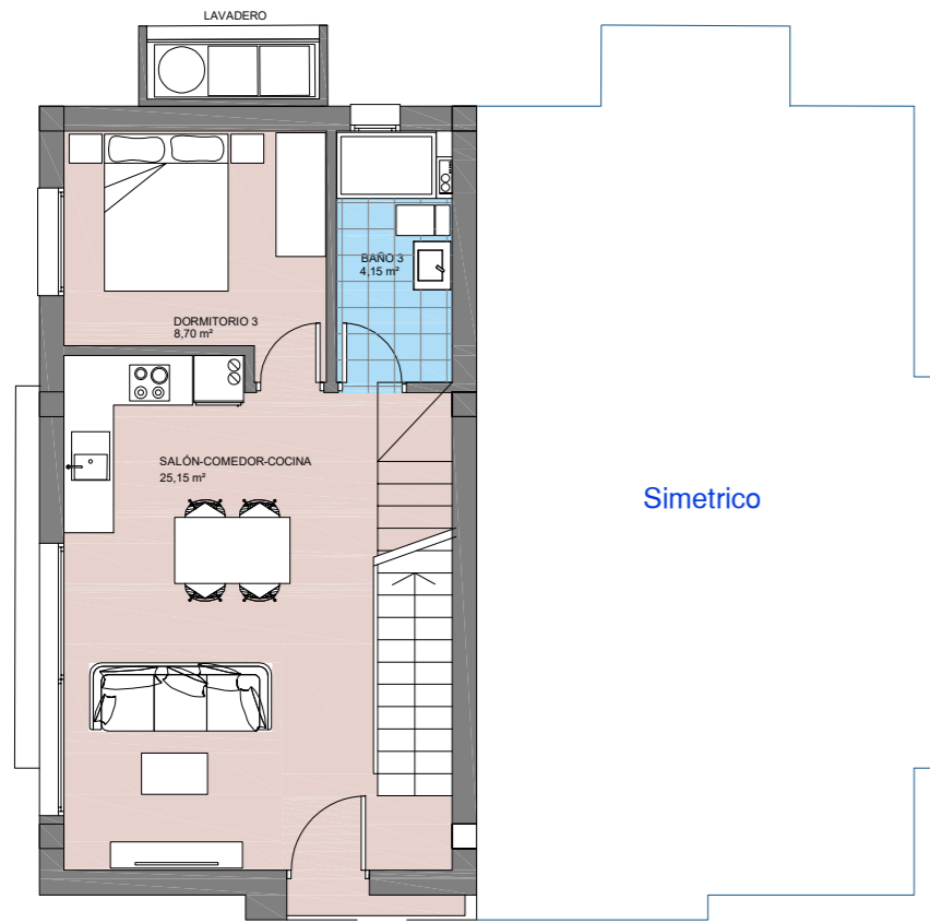
PLANTA BAJA
