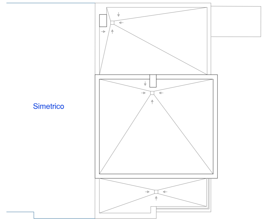
PLANTA CUBIERTA
