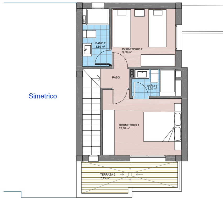
PLANTA PRIMERA
