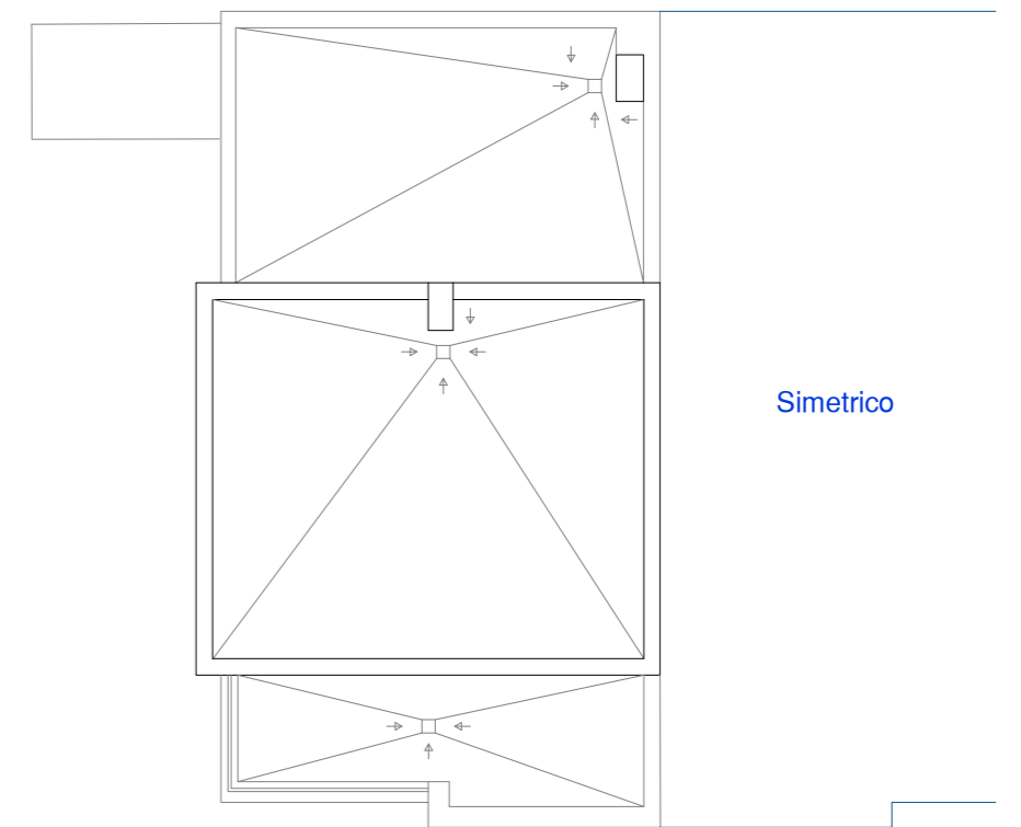
PLANTA CUBIERTA
