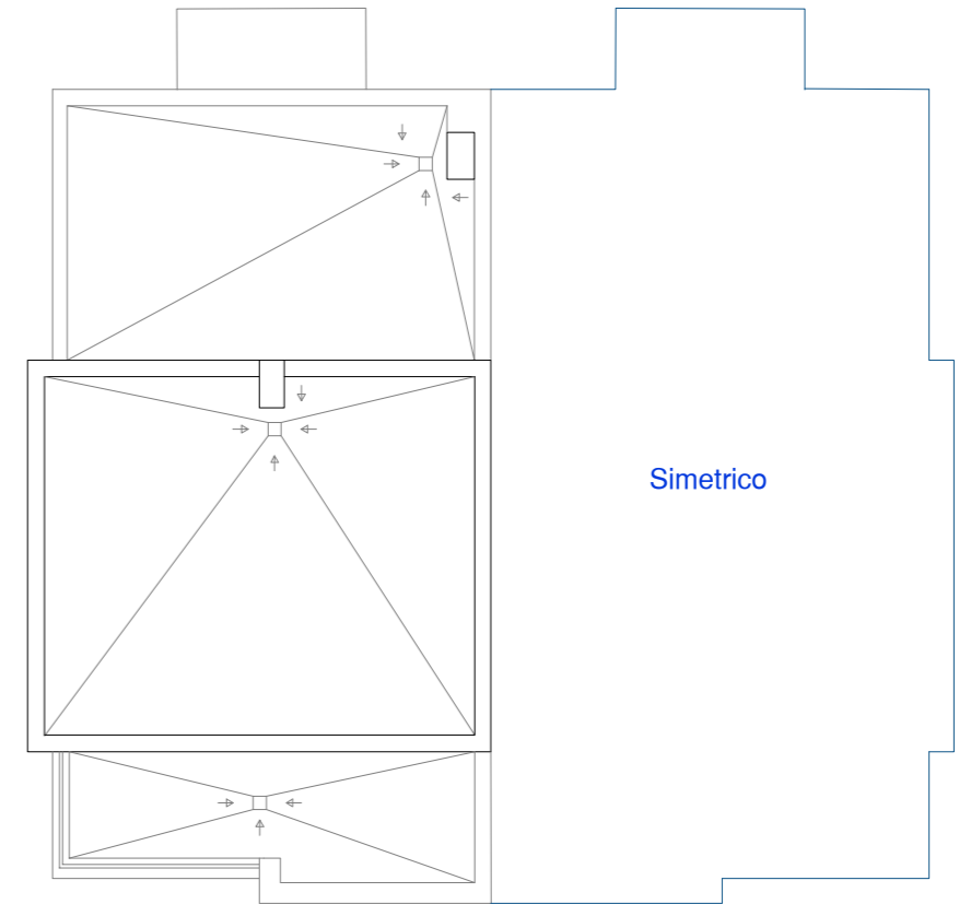
PLANTA CUBIERTA
