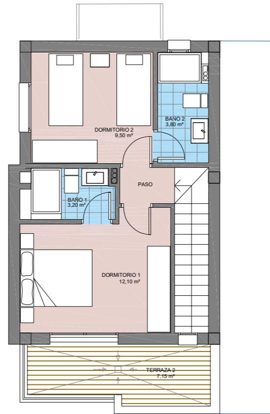
PLANTA PRIMERA
