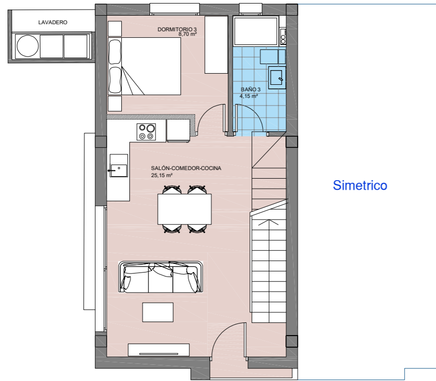
PLANTA BAJA
