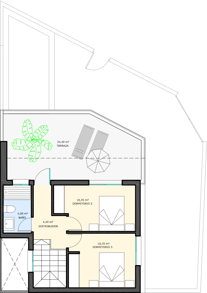
PLANTA PRIMERA
