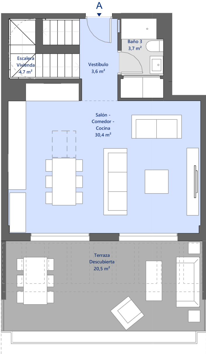
Planta segunda
