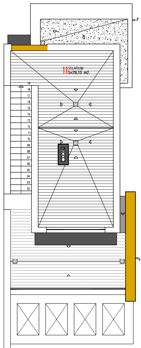
PLANTA SOLARIUM
