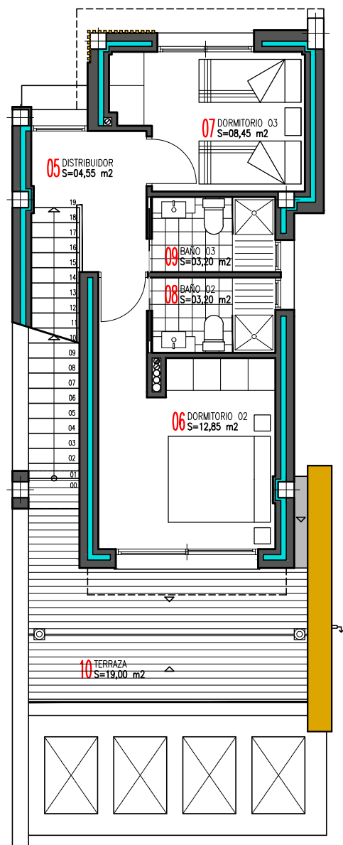
PLANTA PRIMERA
