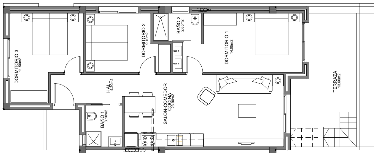
Planta Segunda
