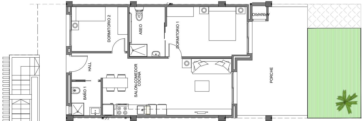
Planta Baja
