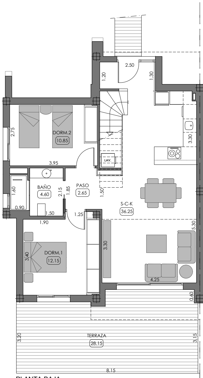
PLANTA BAJA
