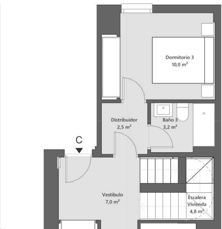
Planta primera
